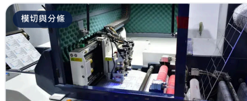
瑞邦 RBJ-350 數位模切機
